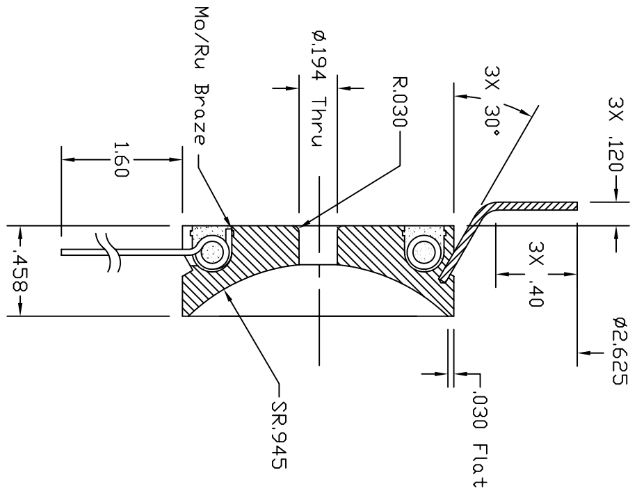
View A-A
